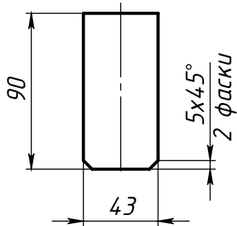
Поз.3 (Ребро среднее)
