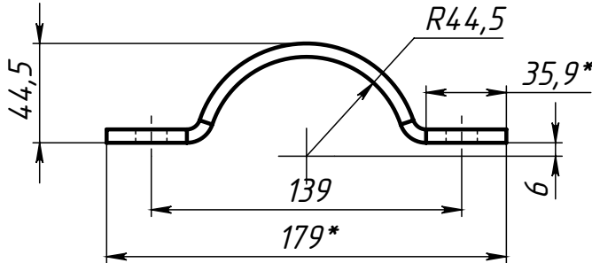
Поз.4 (Полухомут)
